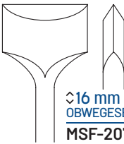
12 mm OBWEGESER 225 mm MSF-206 \angle 1:1
