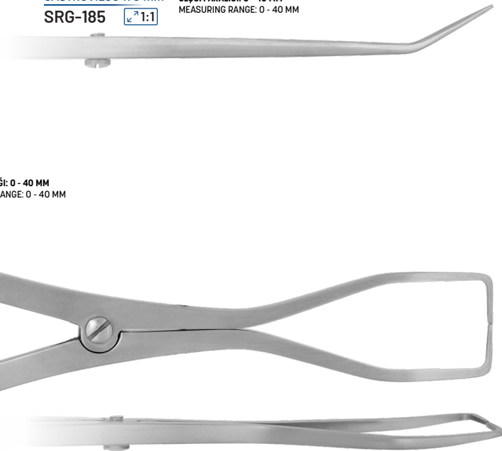
ÖLÇÜM ARALIĞI: 0 - 40 MM MEASURING RANGE: 0 - 40 MM
