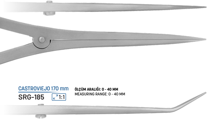
ÖLÇÜM ARALIĞI: 0 - 40 MM MEASURING RANGE: 0 - 40 MM
